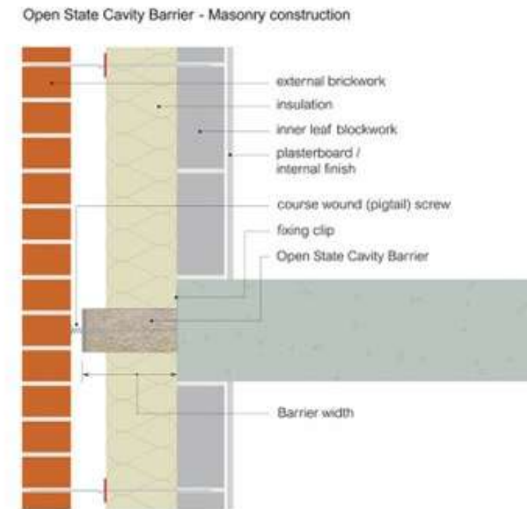
OPEN STATE CAVITY BARRIER - COSTRUZIONE IN MURATURA
