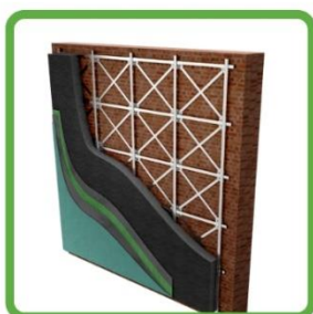
CAPPOTTO ANTISISMICO
